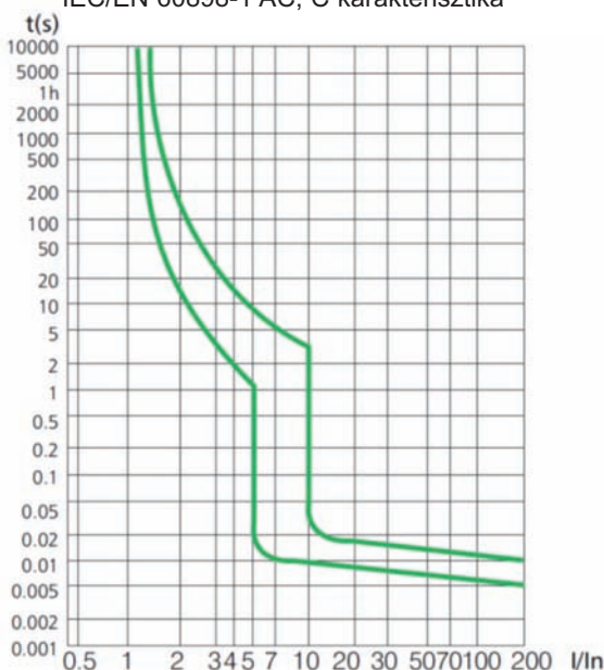
IEC/EN 60898-1 AC, C karakterisztika
