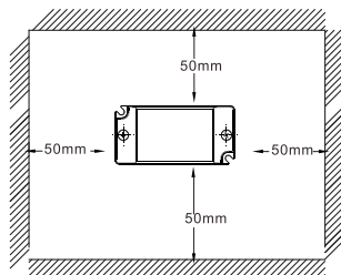
Sugerowany sposób montażu oraz przestrzeń wokół zasilacza
