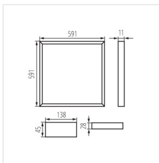
AVAR 6060 32W-CCT
