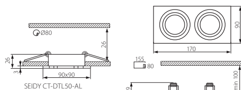
SEIDY CT-DTL50-AL
