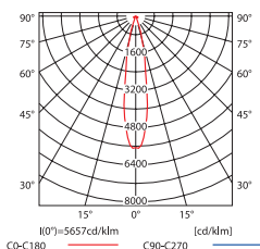
MATEO DLP-150 + AR-111
